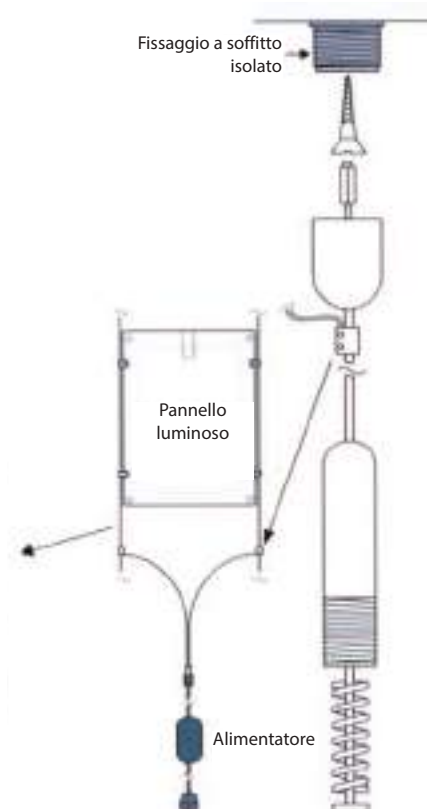
CONNETTORE ALIMENTAZIONE
