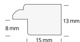
Sezione cornice dimensioni reali Frame section real sizes
