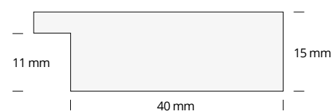
Sezione cornice dimensioni reali Frame section real sizes
